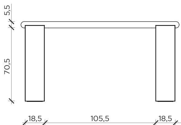
LATO | SIDE
