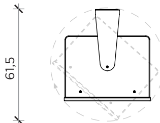
GIREVOLE | SWIVEL
