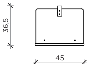
PIANTA | PLAN
